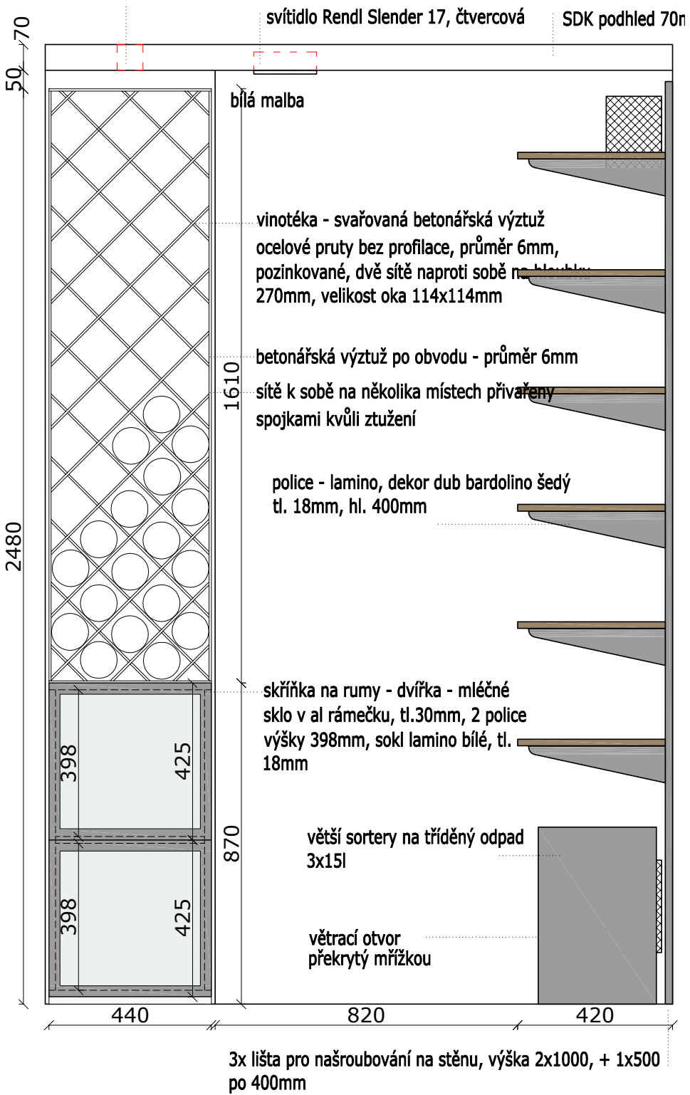
POHLED NA VINOTÉKU - PROVEDENÍ Z BETONÁŘSKÉ VÝZTUŽE (VIZ REFERENCE)
