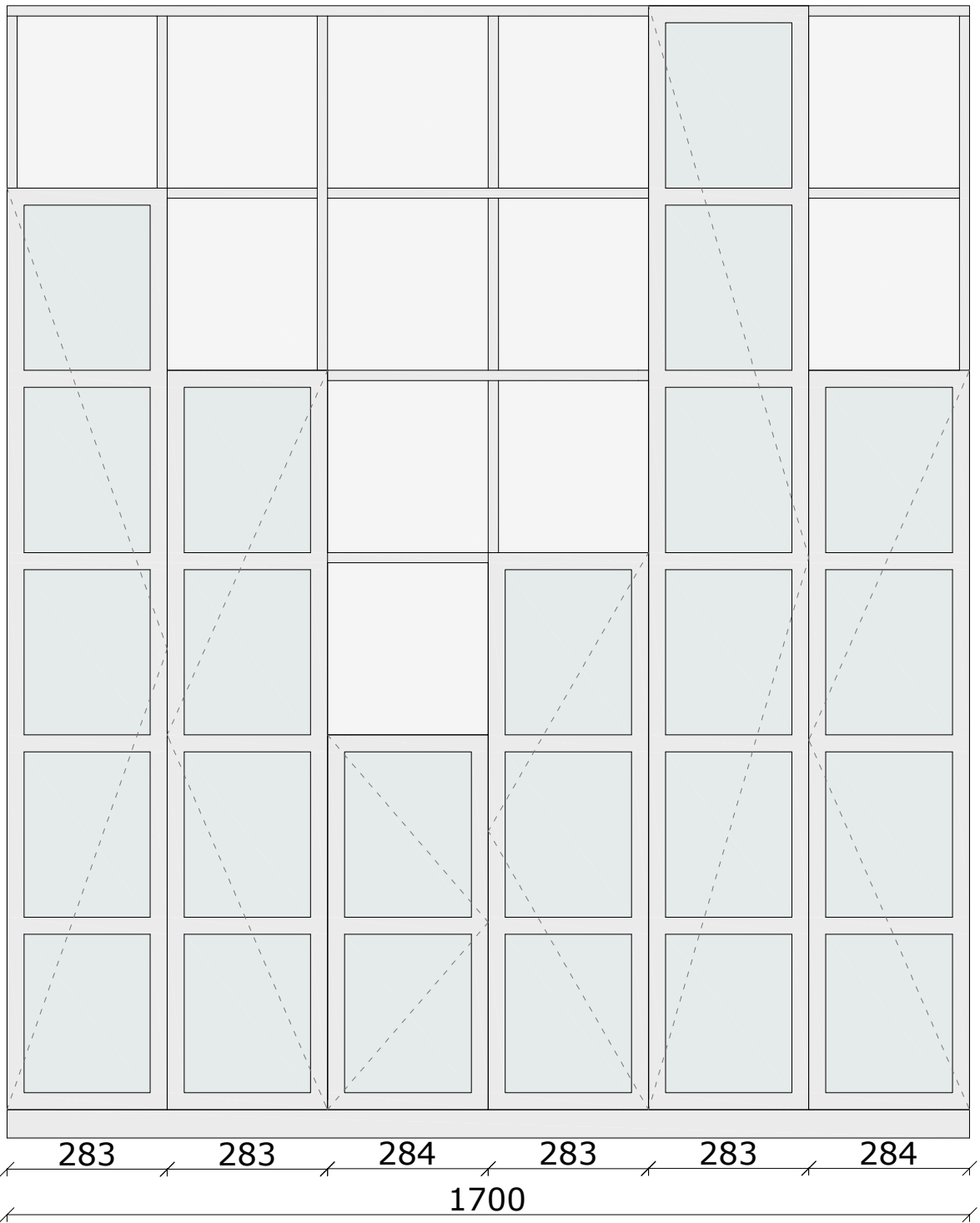
částečně uzavřená knihovna s otevřenými poličkami s bílými zády, hliníkové rámy poliček nastříkané na bílo vyplněné bílým pískovaným sklem, tl. rámů 30mm (typ S5), materiál poliček a zad: bílé lesklé lamino, tl. 18mm, vnitřní police nastavitelná výška
