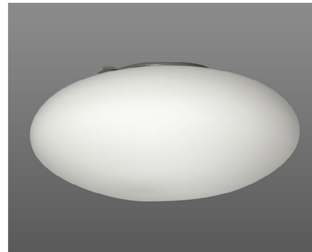
stropní svítidlo Asterion (LUCIS) - prům. 350 mm
