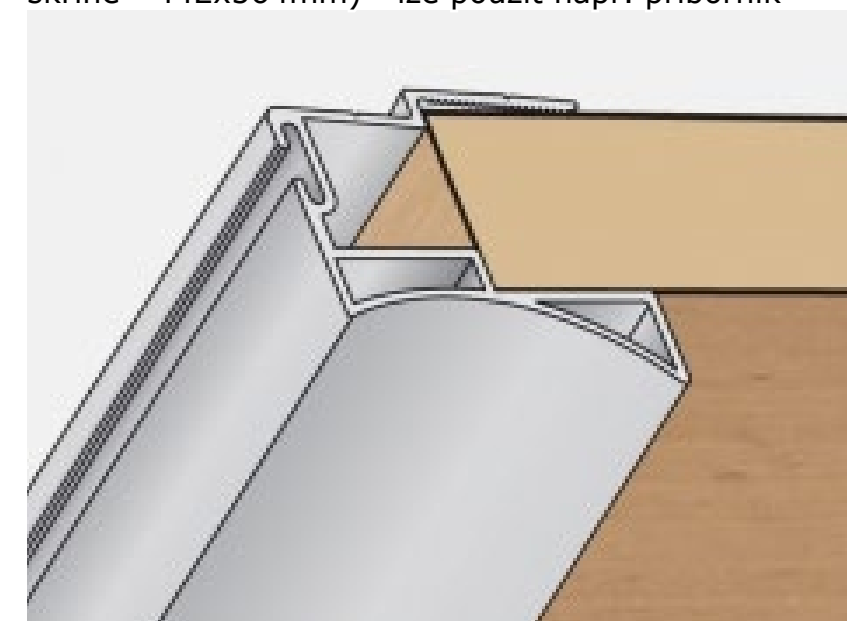
narážecí úchytkový profil - posuvné dveře skříně
