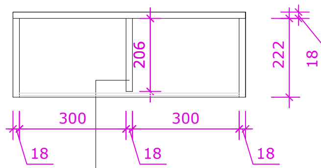
VODOROVNÝ ŘEZ
