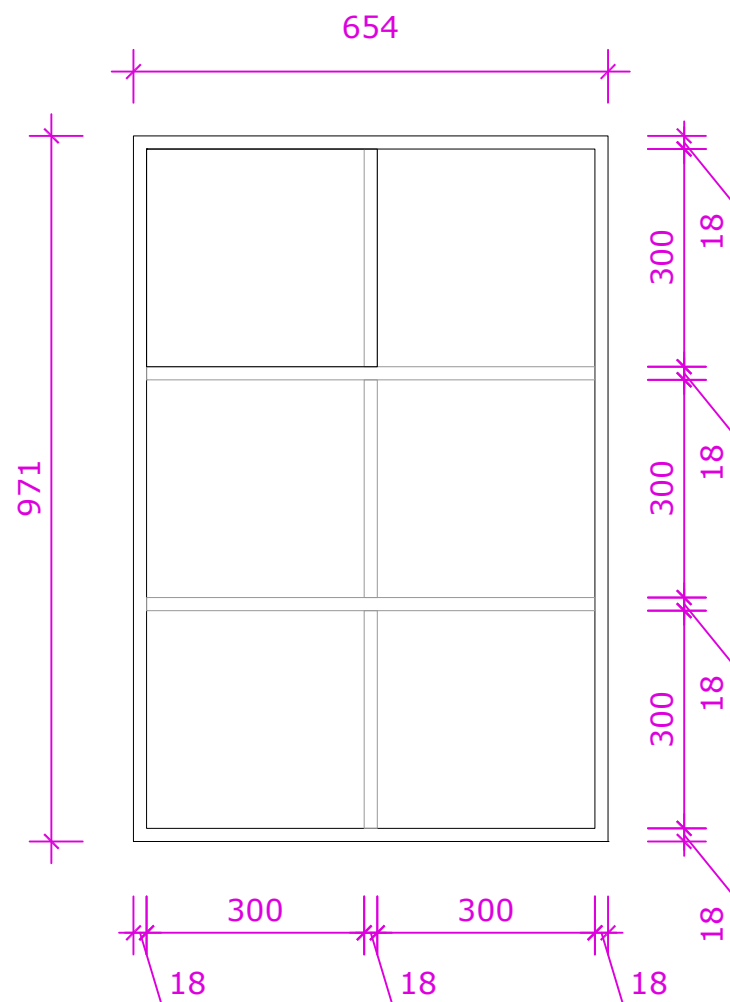
POHLED - KORPUS
