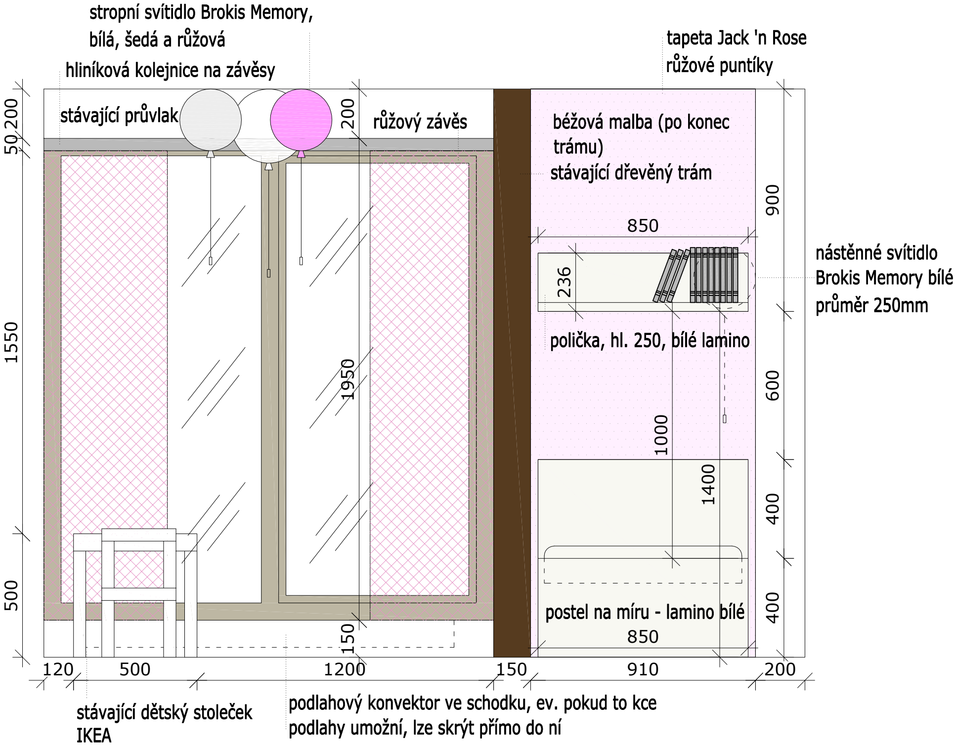
SVÍTIDLA BALONKY BROKIS MEMORY: Bílé svítidlo - průměr 300mm, šedé a světle růžové svítidlo - průměr 250mm
